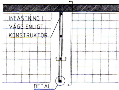
PLAN 1:100
